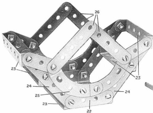
Fig. 4. Vue détaillée de la nacelle
