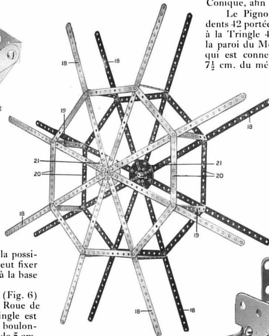
Fig. 5. Détails de la Roue
